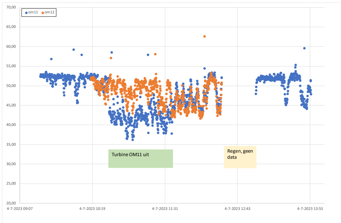
Figuur I.14 Verloop over tijd van de IEC-meting bij OM11 en de langdurende indicatieve meting bij OM12
