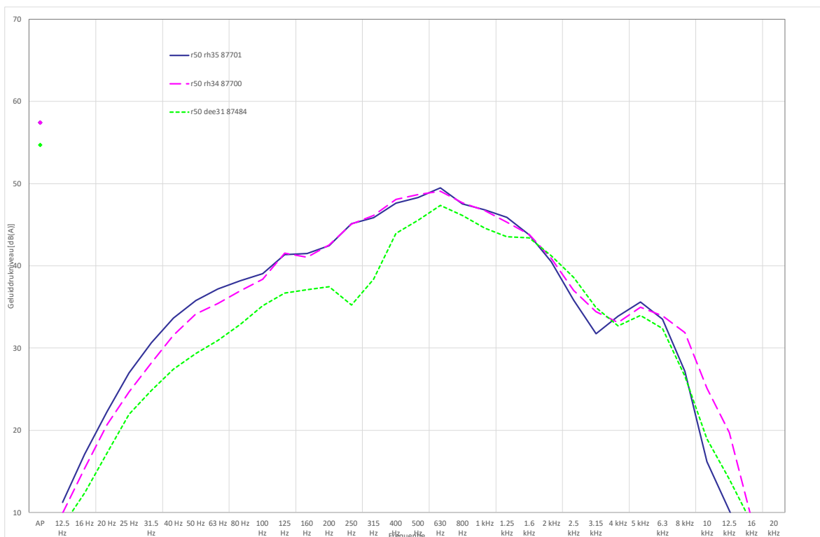
Figuur I.15 Spectrum kortdurende indicatieve metingen 11 oktober 2023
